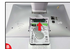
Vložte SATA disk.
